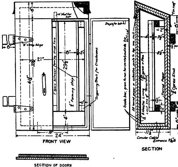
FIG. 117.—Cable box.
